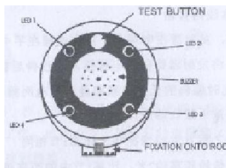
图 3 型数字无线核相器发射器底座
